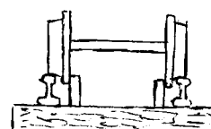
NORMÁL NYOMTÁVÚ JÁRMŰ (A TERELEST A BELSŐ TERELELŐ VÉGZI)
