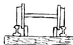
NORMÁL NYOMTÁVÚ JÁRMŰ (A TERELEST A BELSŐ TERELELŐ VÉGZI)
