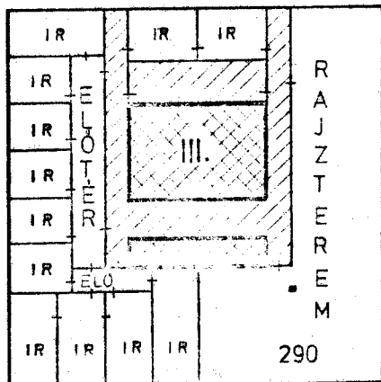
AZ alaprajz egy-egy korábbi elgondolást mutat, csak tájékoztatásként közöljük!
